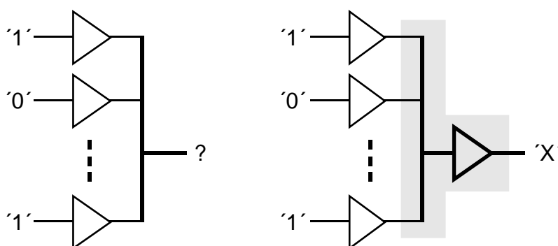
Abb. B-20: Wirkung von Auflösungsfunktionen
