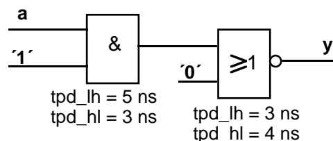
Abb. B-17: Flankenabhängige Laufzeiten
